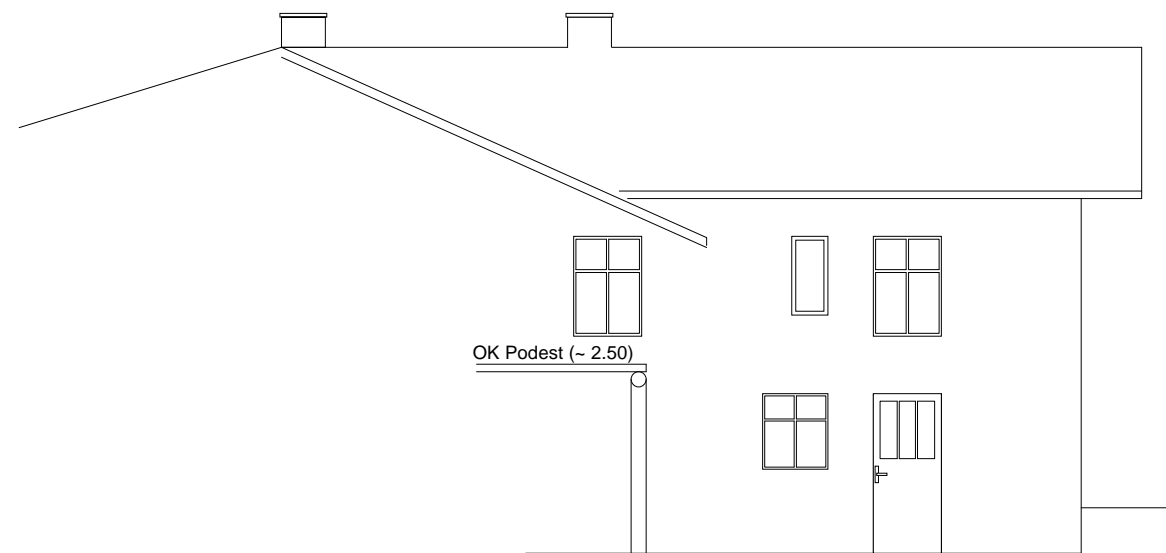
Ansicht Südost M= 1:100
